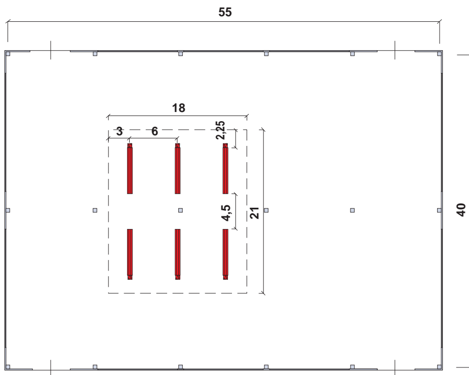
Fig. 16 Esquema de instalación para la calefacción de un área parcial
