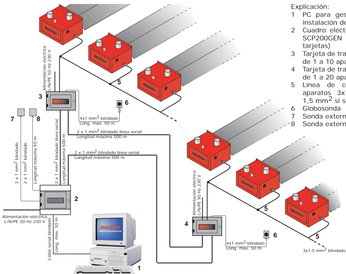
Fig. 44 Conexión eléctrica con cable de 2 conductores
