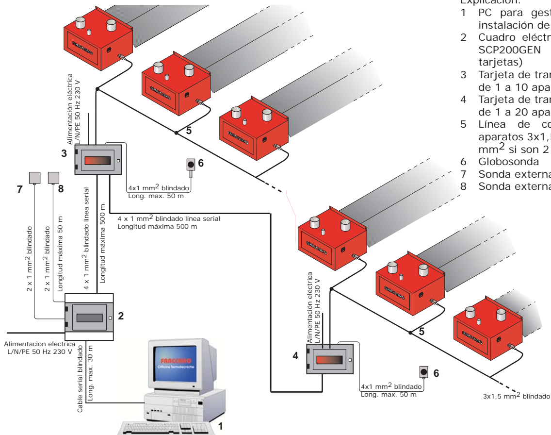
Fig. 45 Conexión eléctrica con cable de 4 conductores
